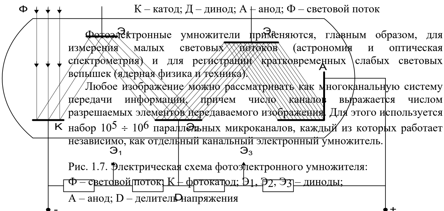
Рис.1.7. Электрическая схема фотоэлектронного умножителя.
