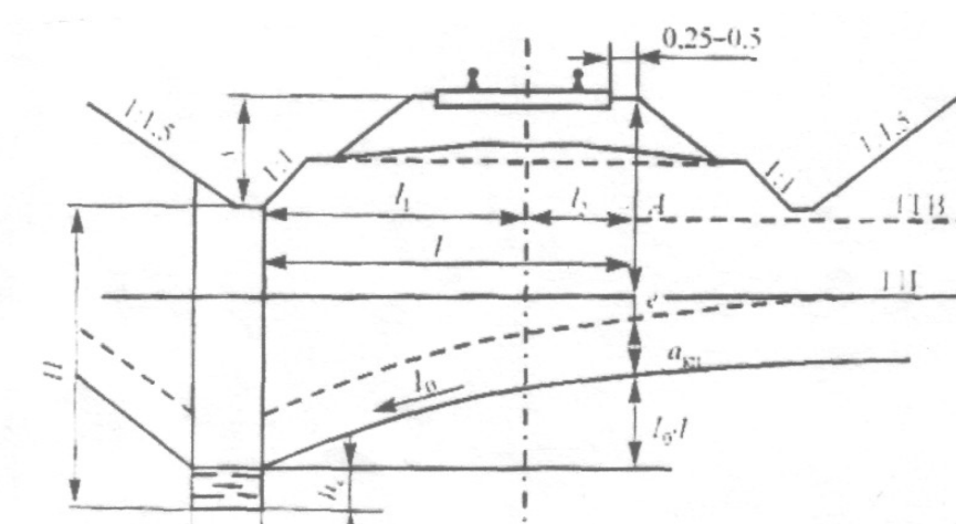
Рис. 3.1 Схема одностороннего подкюветного дренажа
