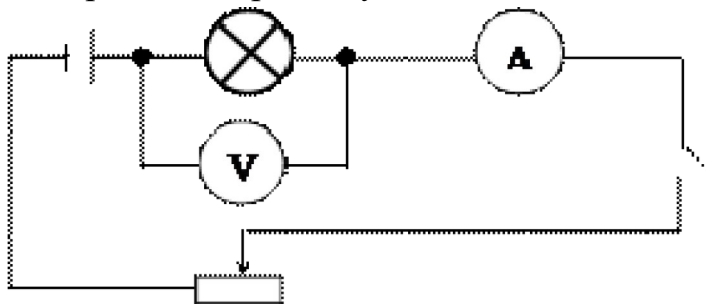
Рис. 2. Схема установки
