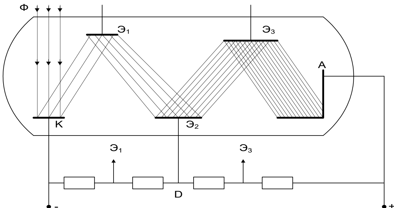
Рис.1.7. Электрическая схема фотоэлектронного умножителя. \Phi - световой поток; К - фотокатод; Э 1 , Э 2 , Э 3 - диноды; А - анод; D - делитель напряжения
