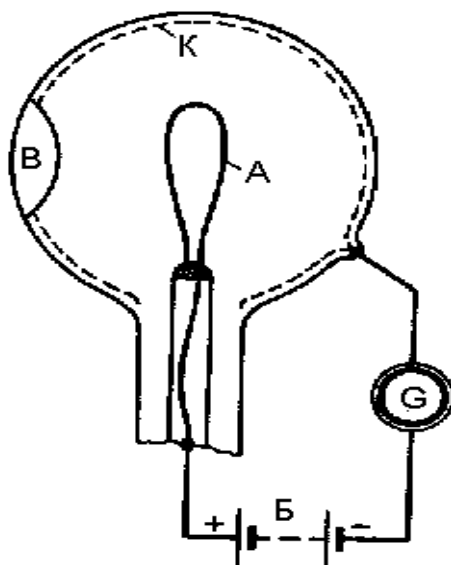
Рис. 1.5. Устройство фотоэлемента и схема его включения в цепь.
