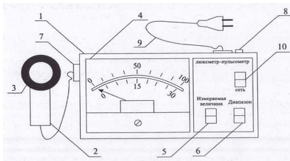
Рис. 2. Внешний вид люксометра-пульсметра «БЖшМ»
