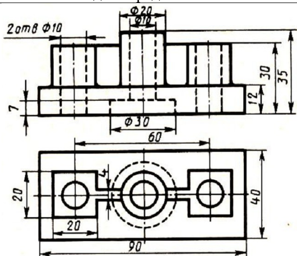
Опора
