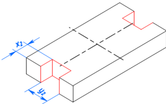
Изображение призматического паза в основании
