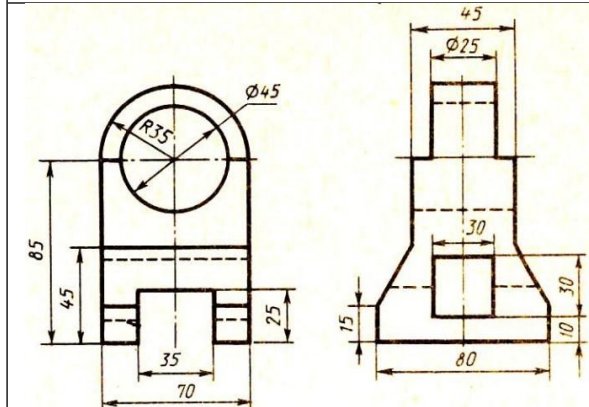
Кронштейн
