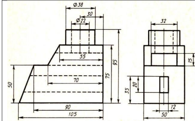
Корпус
