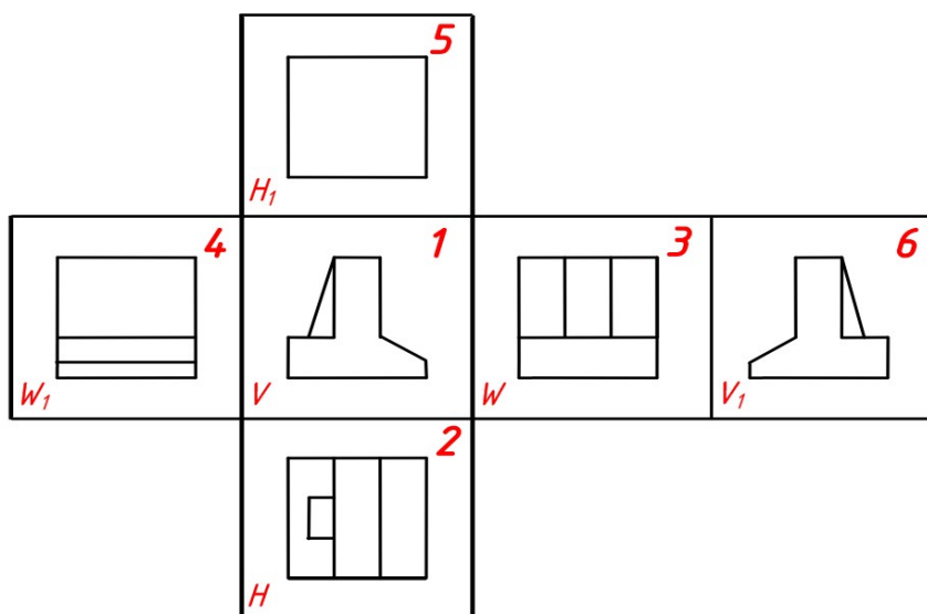
Рисунок 3 Основные виды
