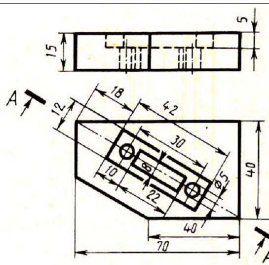
Плита
