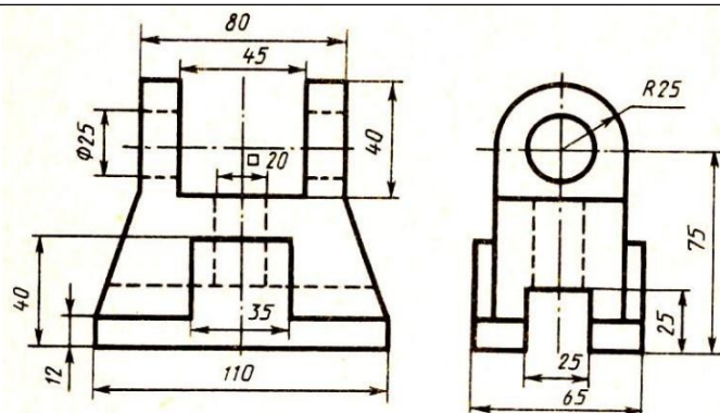
Кронштейн
