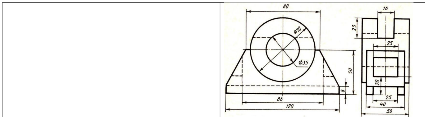
Стойка
