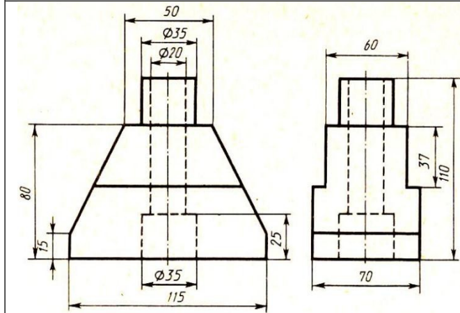
Станина
