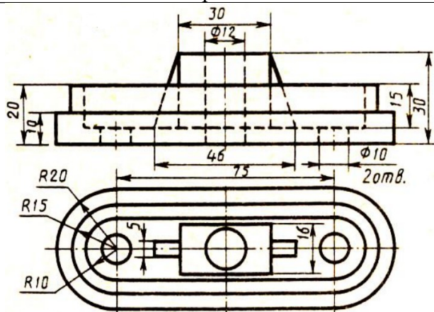
Onopa
