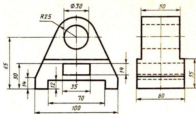
Стойка
