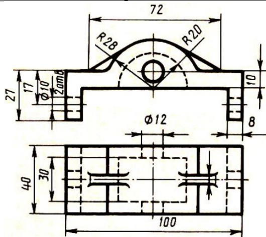
Корпус
