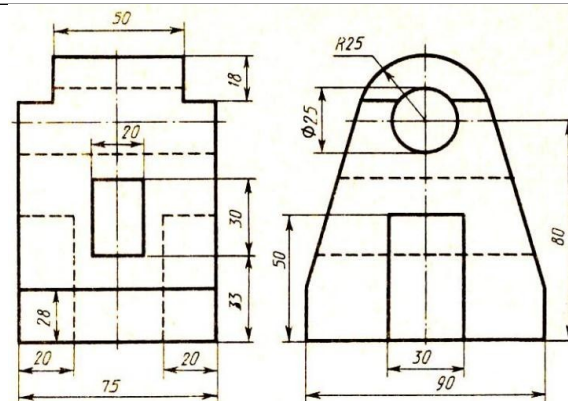
Стойка
