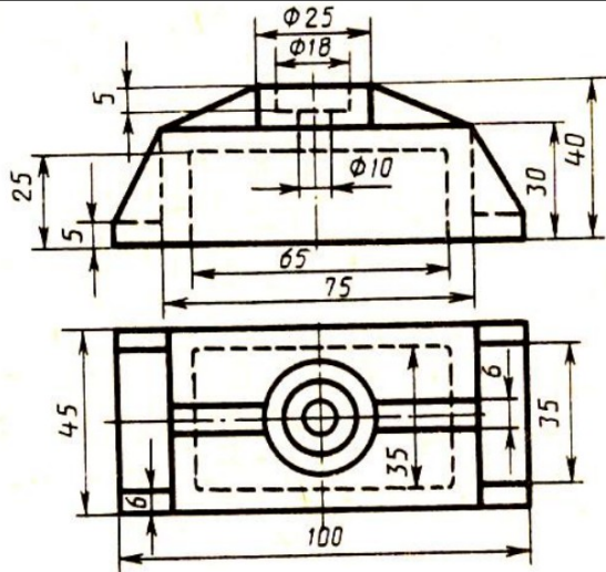
Крышка
