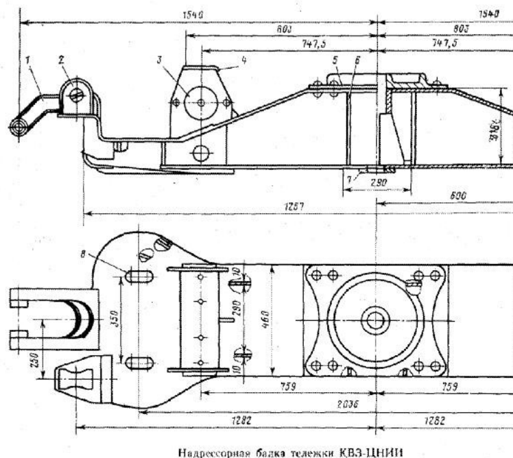
Надрессорная балка тележки КВЗ-ЦНИИ 1
