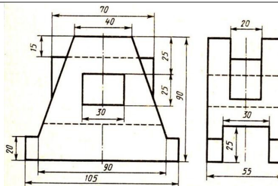
Станина
