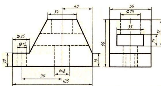
Onopa
