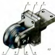
Рисунок 1 Сборочный узел «Блок направляющий»
