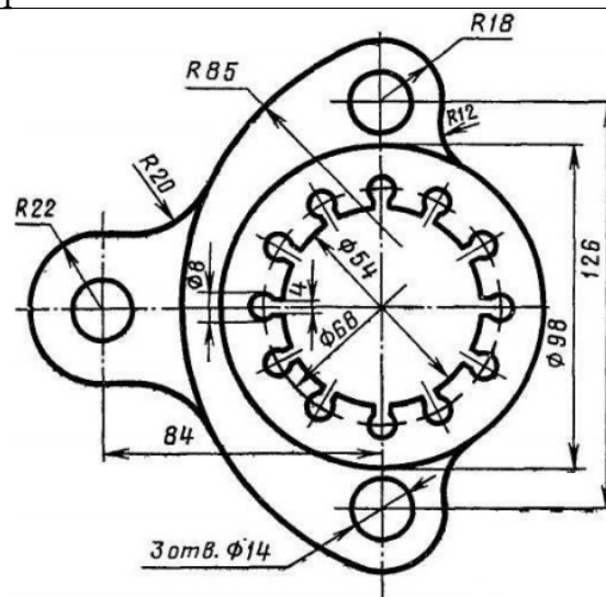
Розетка
