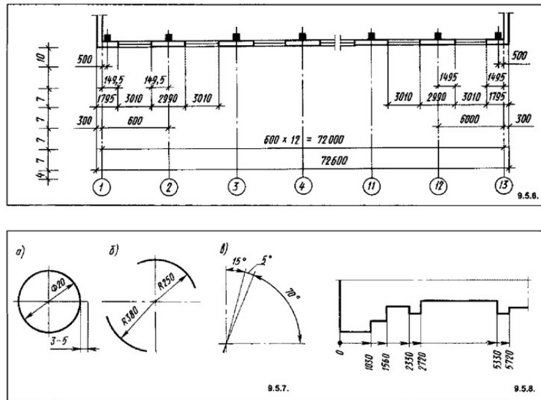
Рисунок 3 Нанесение отметок
