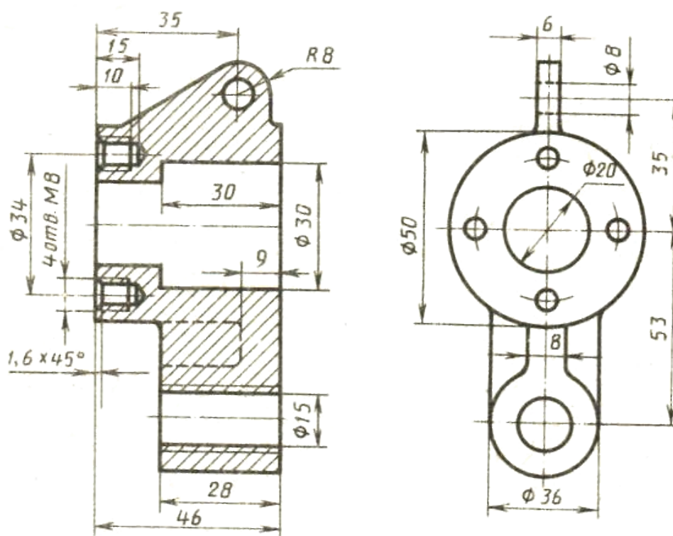
Подвеска
