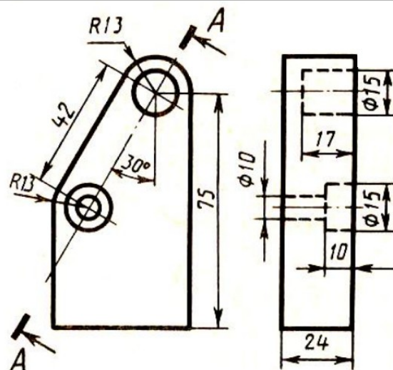
Планка
