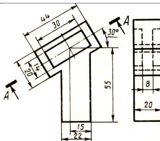
Пластина
