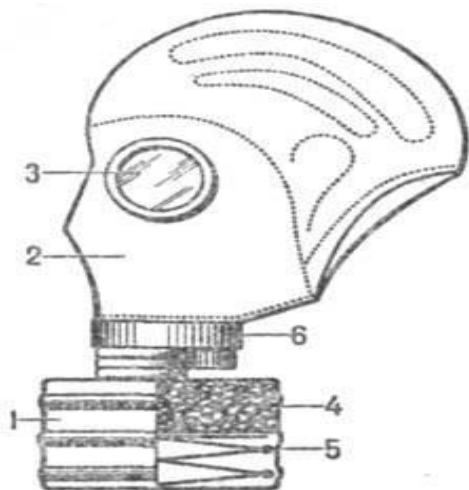
Рис. 1. Фильтрующий противогаз
