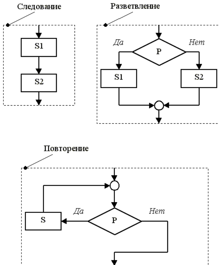
Рис. 1. Основные управляющие конструкции структурного программирования. Основными конструкциями структурного программирования являются: следование,
