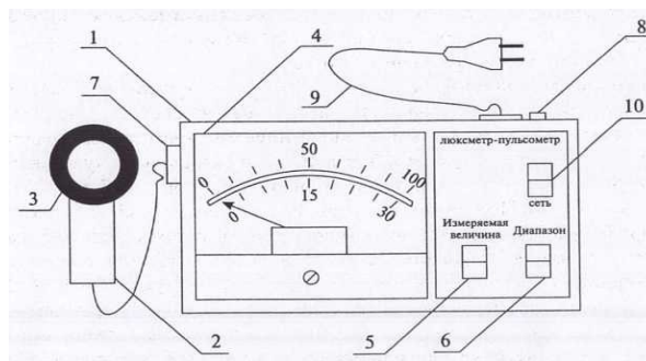
Рис. 2. Внешний вид люксметра-пульсметра «БЖШМ»
