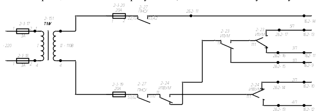
Рисунок 3.1 - Принципиальная схема
