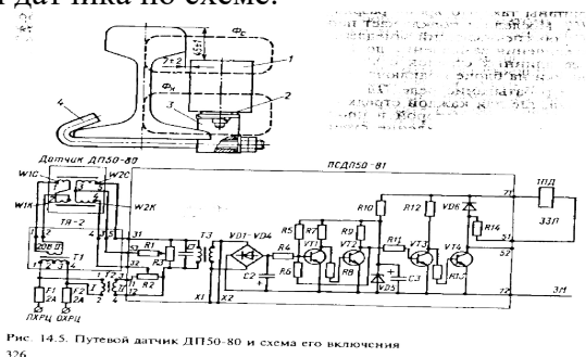
Рис. 14.5. Путевой датчик ДП50-80 и схема его включения
