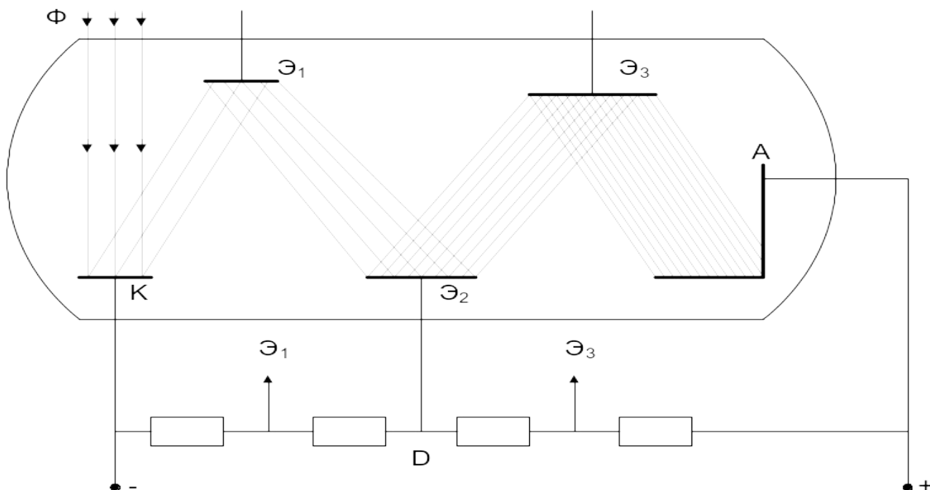
Рис.1.7. Электрическая схема фотоэлектронного умножителя. \Phi - световой поток; К - фотокатод; \mathcal{E}_1, \mathcal{E}_2, \mathcal{E}_3 - диноды; А - анод; D - делитель напряжения
