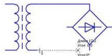
Рисунок 10.7 – Соединение трансформатора и диодного моста
