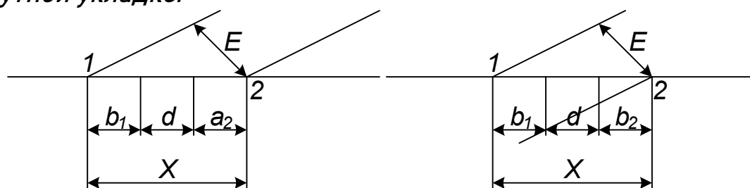
Рисунок 6 Схемы взаимного расположения двух стрелочных переводов.
