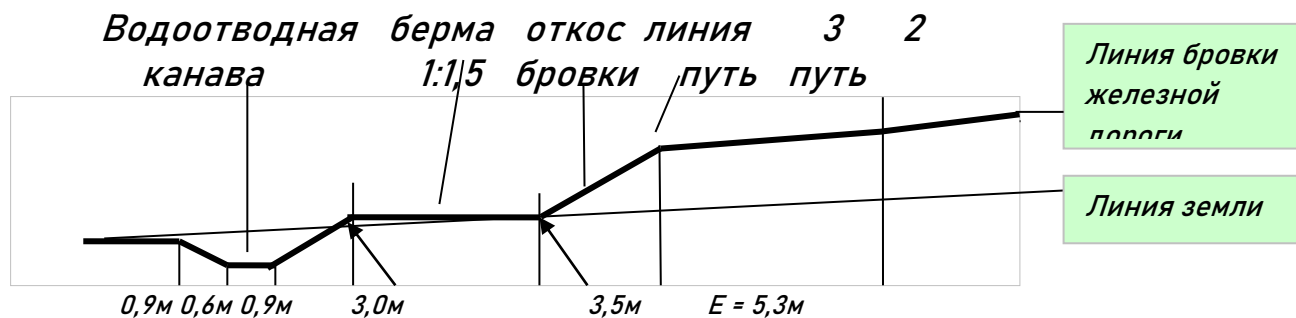
Рисунок 6 Часть поперечного профиля
