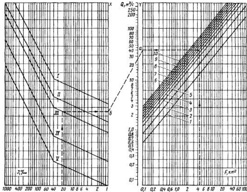
Рис. 5.8. Номограмма для определения расходов дождей паводков вероятности превышения 1 % при песчаных и супесчаных почвах
