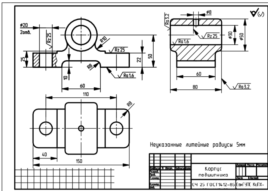
Рисунок 10 Эскиз детали
