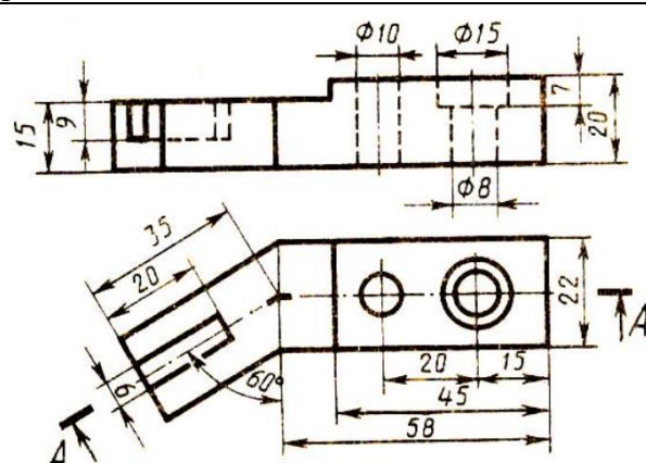
Скоба
