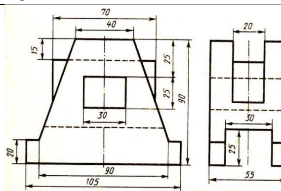
Станина
