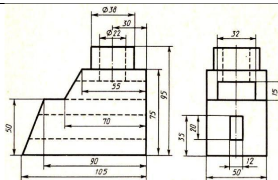
Корпус
