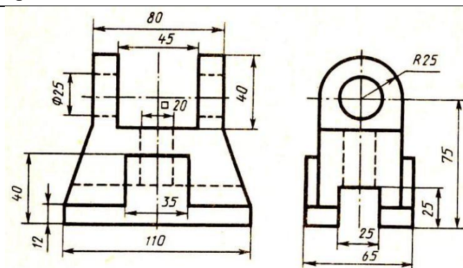
Кронштейн
