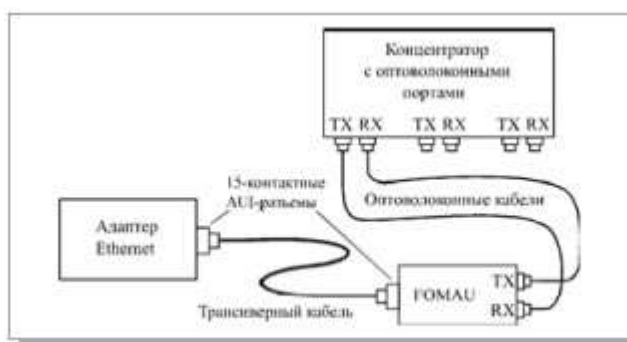
Рисунок 7 – Соединение адаптера и концентратора в 10BASE-FL
